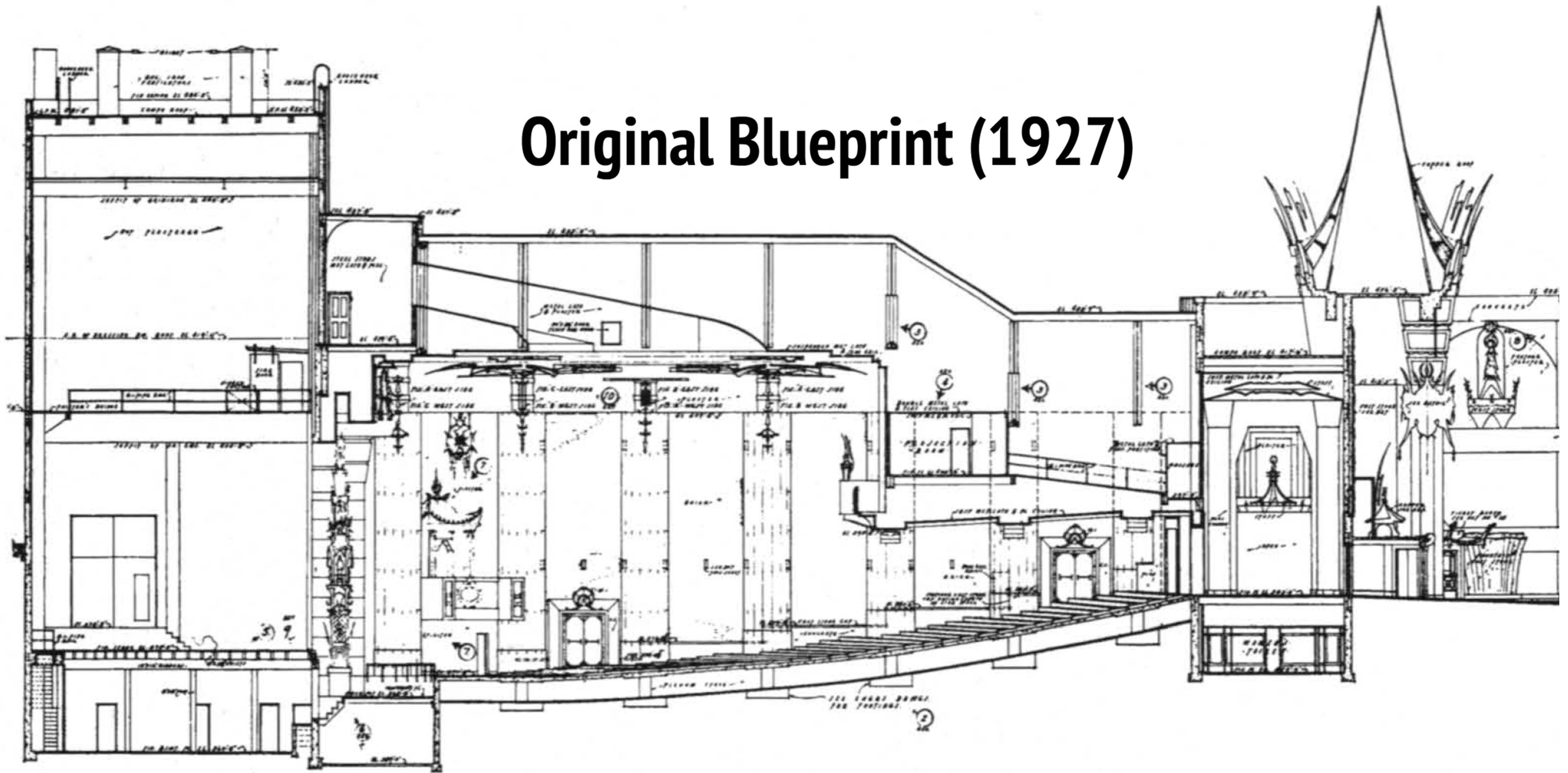
LONGITUDINAL SECTION
